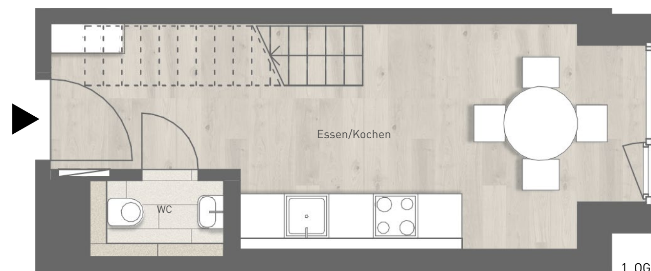
1. OG
