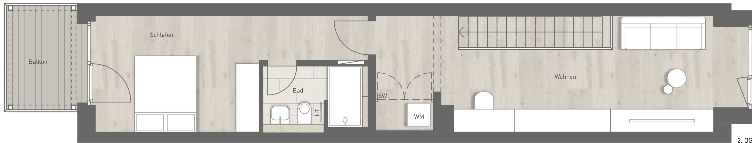
2. OG
